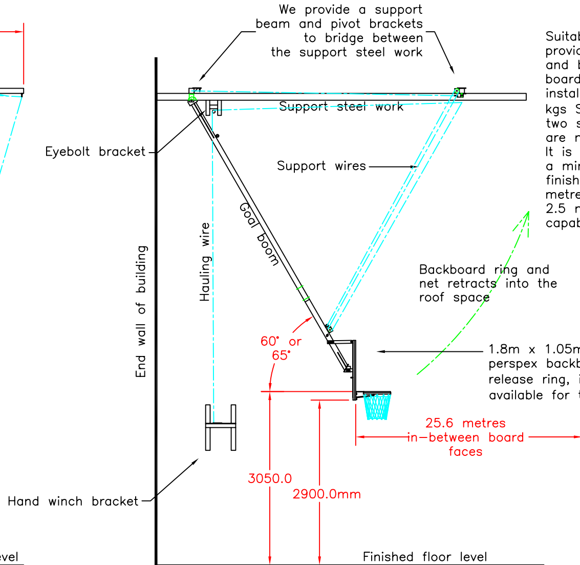
END ELEVATION
